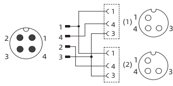
Y2 电路示意图
