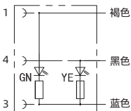
M8母插带两个灯PNP信号接线图
