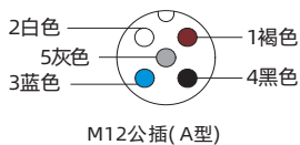
M12公插(A型)
