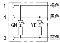
M2母插带两个灯PNP信号接线图
