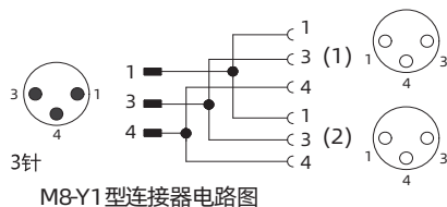
电路示意图
