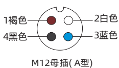
M12母插(A型)
