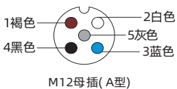
M12母插(A型)
