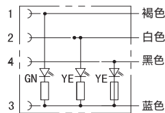
M2母插带三个灯PNP信号接线图
