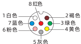
M12母插(A型)
