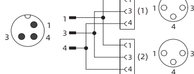
Y1 电路示意图
