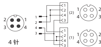
Y3 电路示意图
