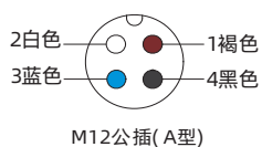
M12公插(A型)
