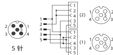
Y3 电路示意图
