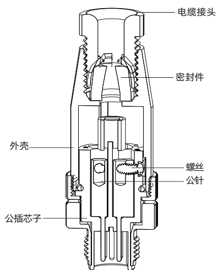
M12直型公连接器
