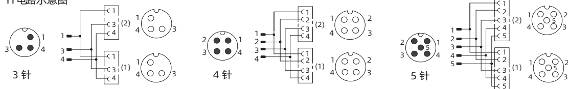
Y1 电路示意图
