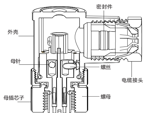
M12弯型母连接器
