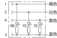
M2母插带三个灯PNP信号接线图
