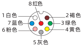
M12母插(A型)
