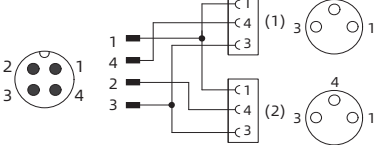
Y2 电路示意图
