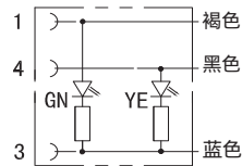
M2母插带两个灯PNP信号接线图
