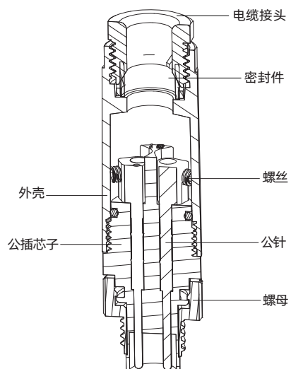
M8直型公连接器
