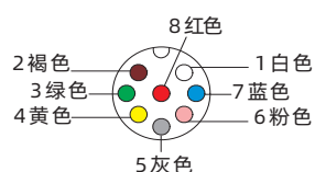
M12公插(A型)
